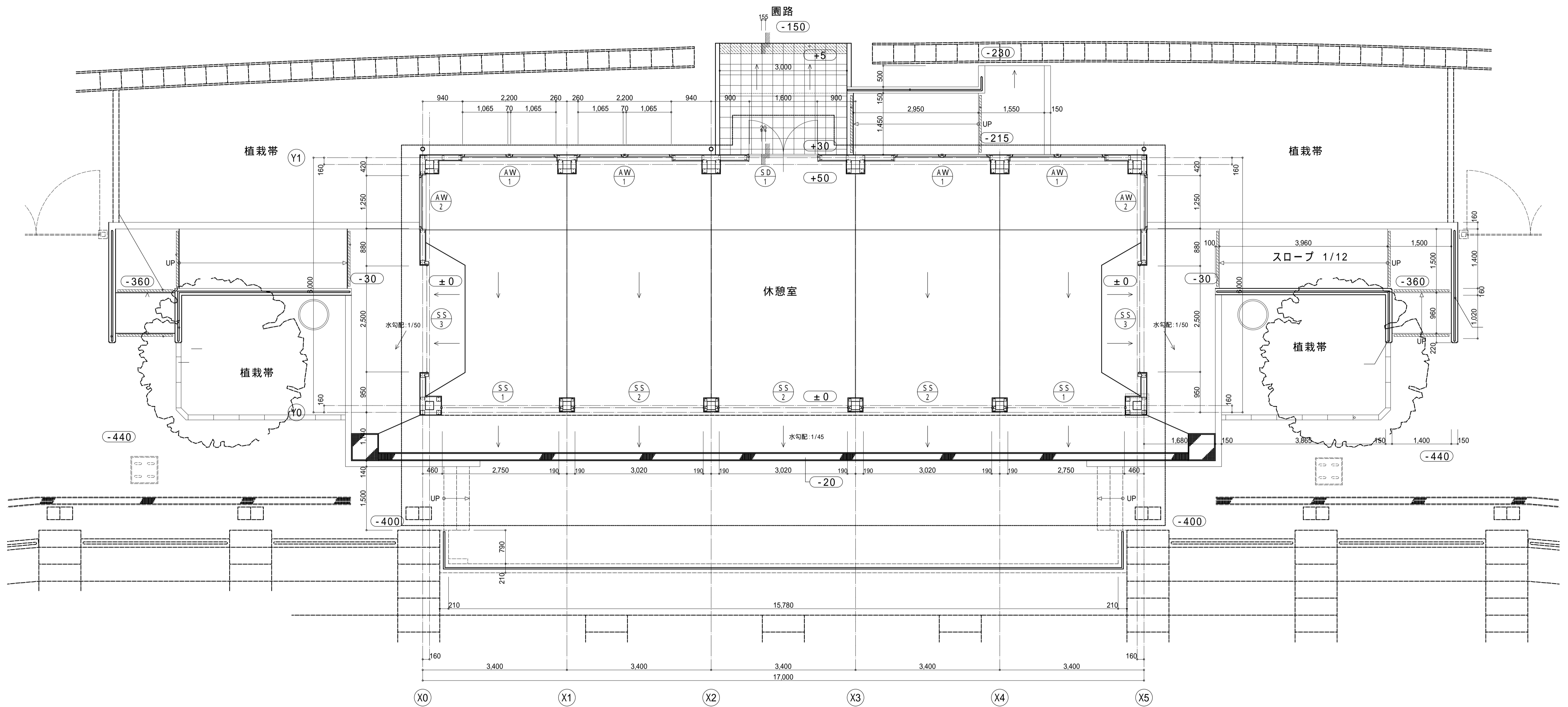
休憩室配置兼平面図 S=1/50
