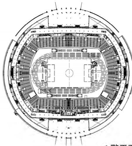
4階平面図
