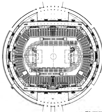
4階平面図
