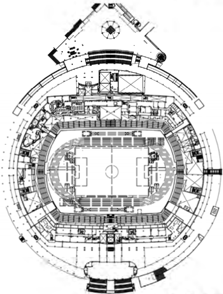
3階平面図
