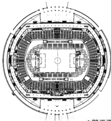
4階平面図
