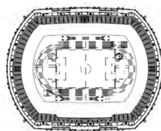
7階平面図
