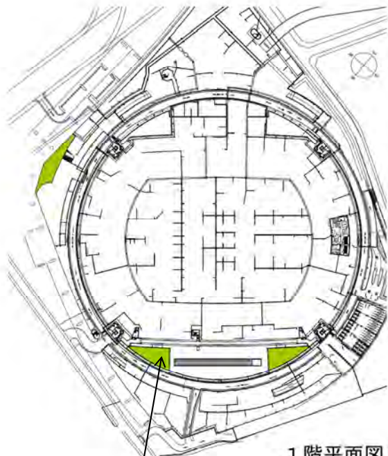
1階平面図
