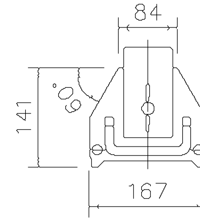
上面図
