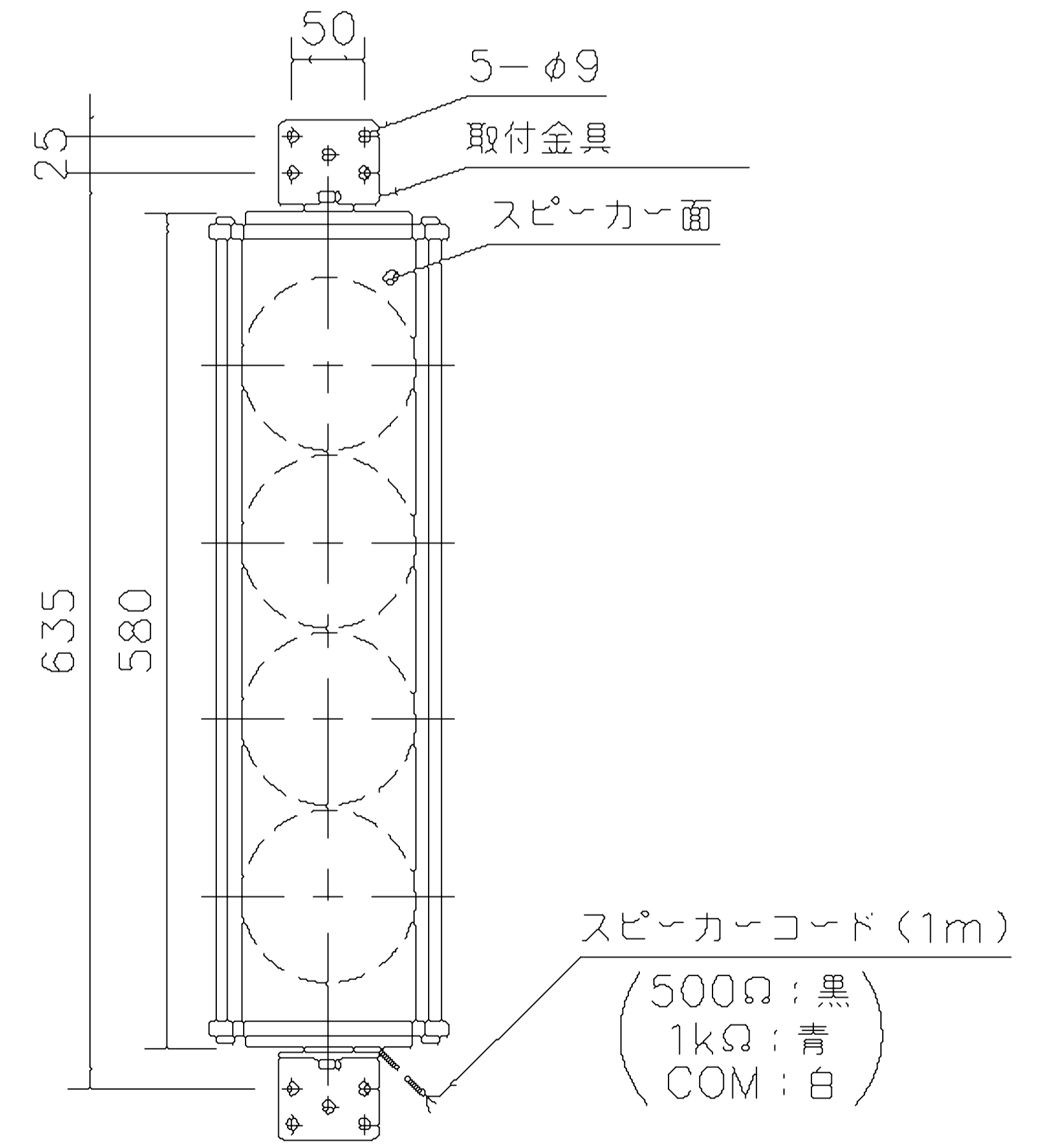
正面図
