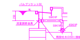
○-○ 配管断面図 (改修後) S=1/20
