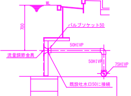
○-○ 配管断面図 (改修後) S=1/20
