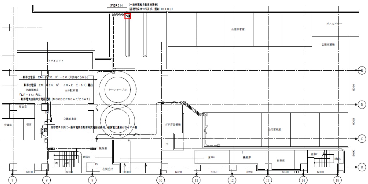
駐車場平面図（既設充電設備設置場所）
