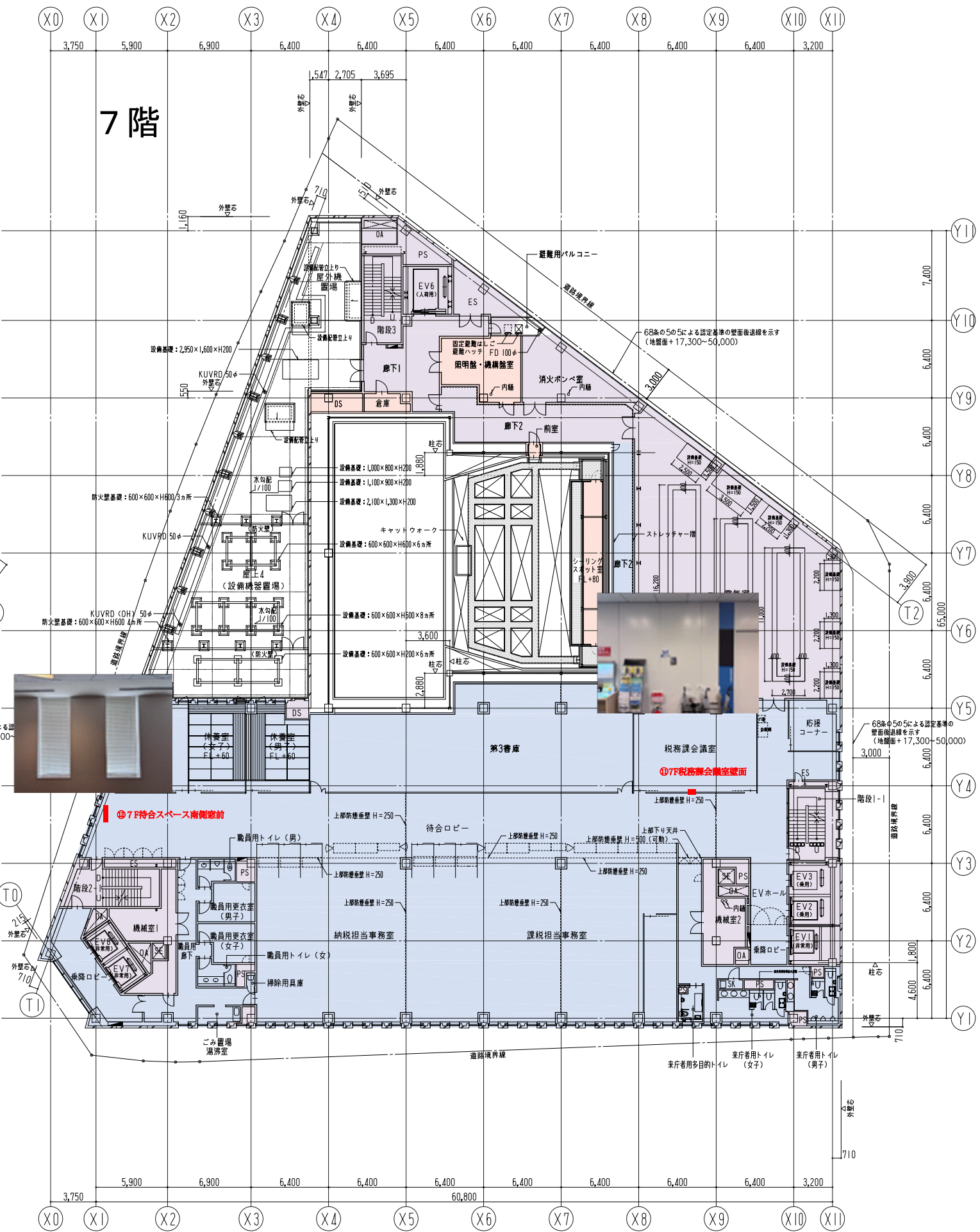
7階平面図 (31Mを超える階)
