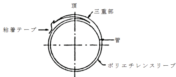
図－３ 直部での固定方法
