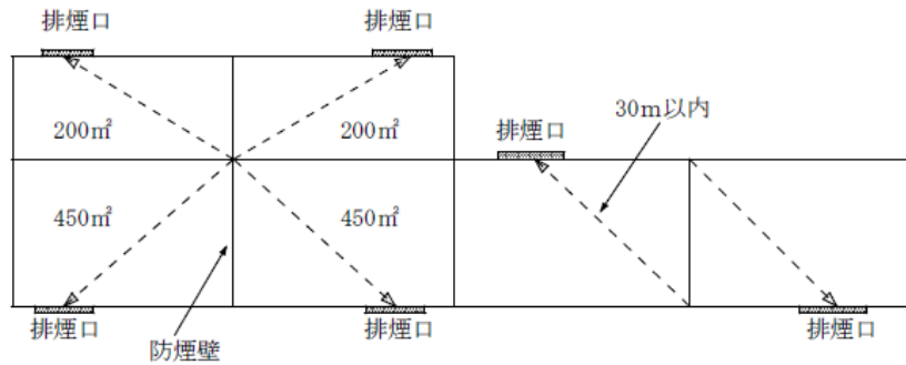
直接外気に接する排煙口
