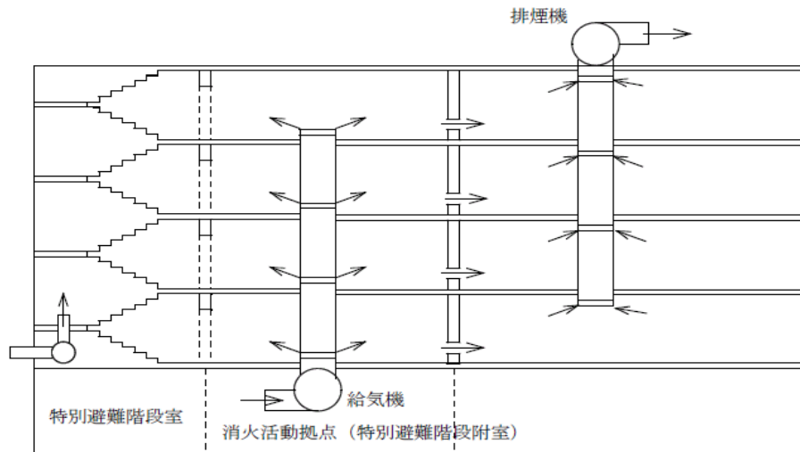
第 18－5 図 消火活動拠点に排煙口を設けない場合（加圧排煙）の例
