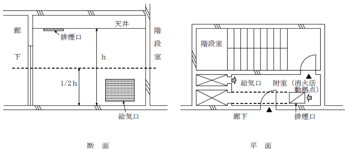
第 18-4 図 消火活動拠点に排煙口を設ける場合の例
