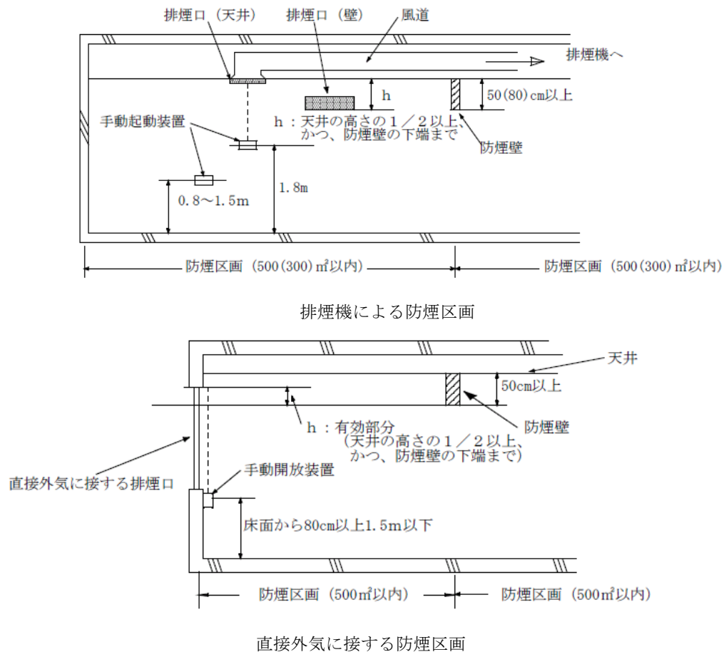
第 18－2 図 防煙区画の断面
