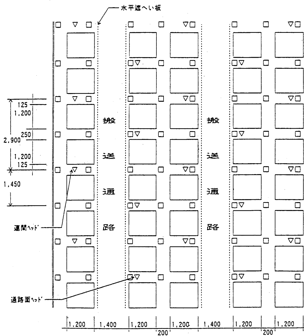
平面 (水平遮へい板直下ーレベル2、4配置)
