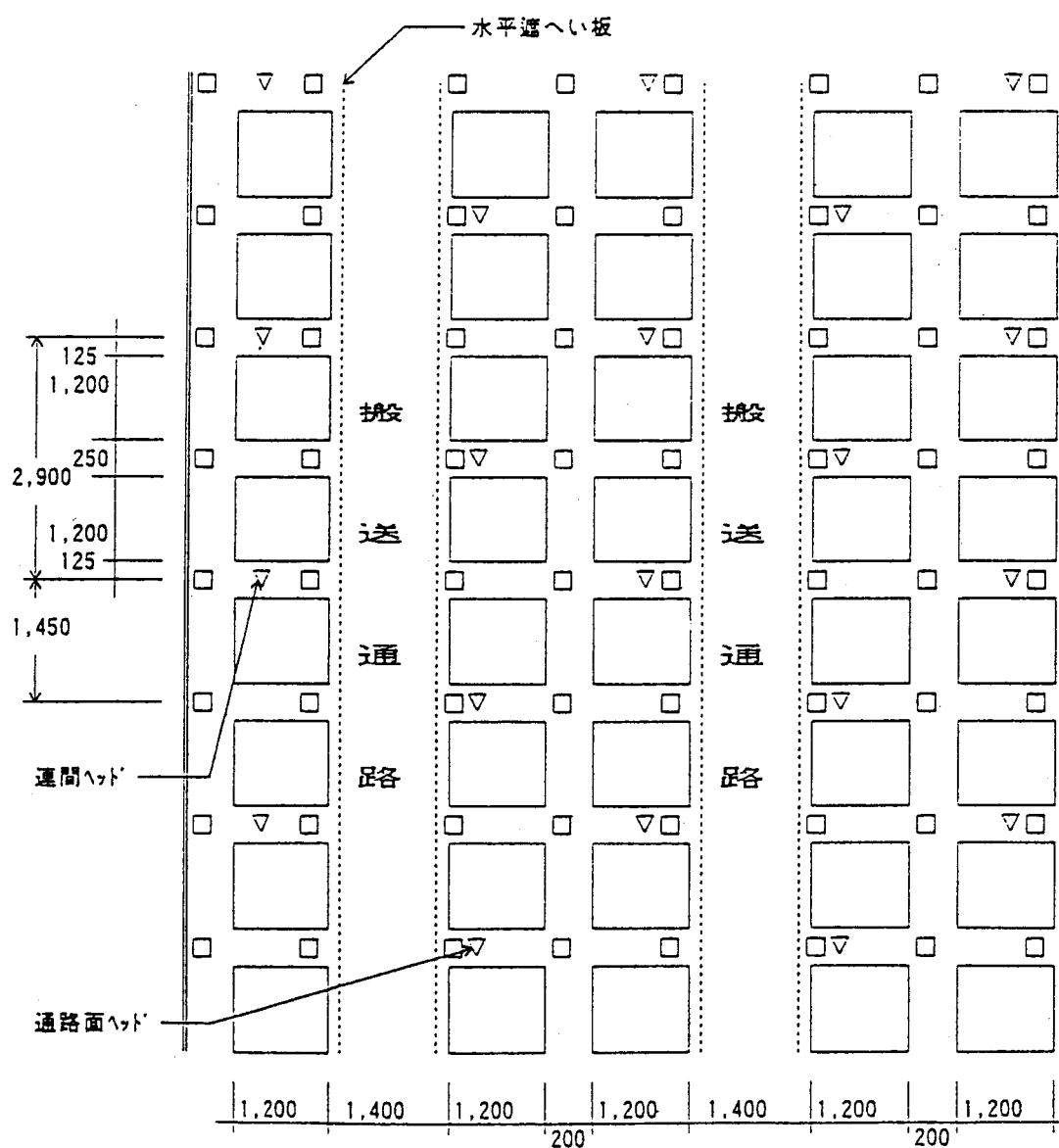
平面 (水平遮へい板直下ーレベル2、4、6配置)
