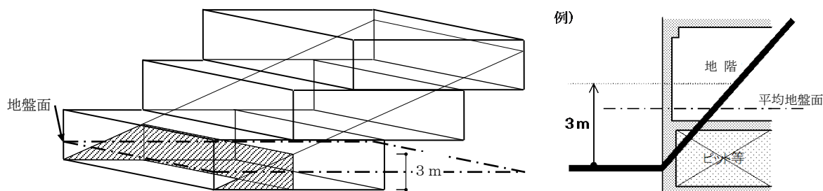
図 2 法第 52 条第 5 項の地盤面
