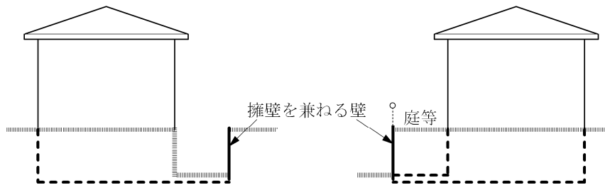
図1 擁壁を兼ねる壁の例
