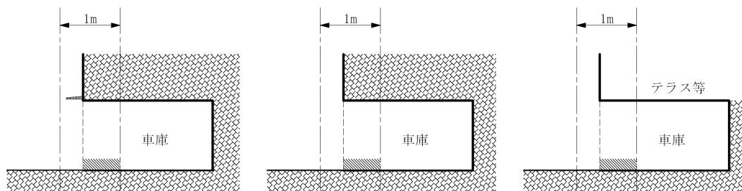
図2 令第135条の21第2号における床面
