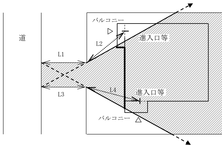
図1 「道から非常用進入口等までの延長が20m以下」及び「バルコニーのその他これらに類するもの位置」
