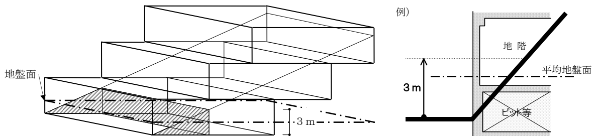
図 2 法 52 条第 5 項の地盤面
