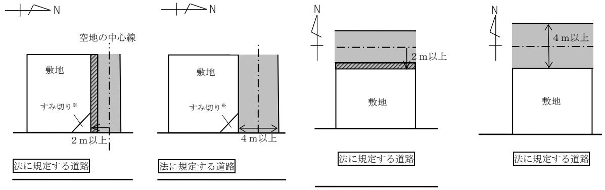
図 1 角敷地の場合①
