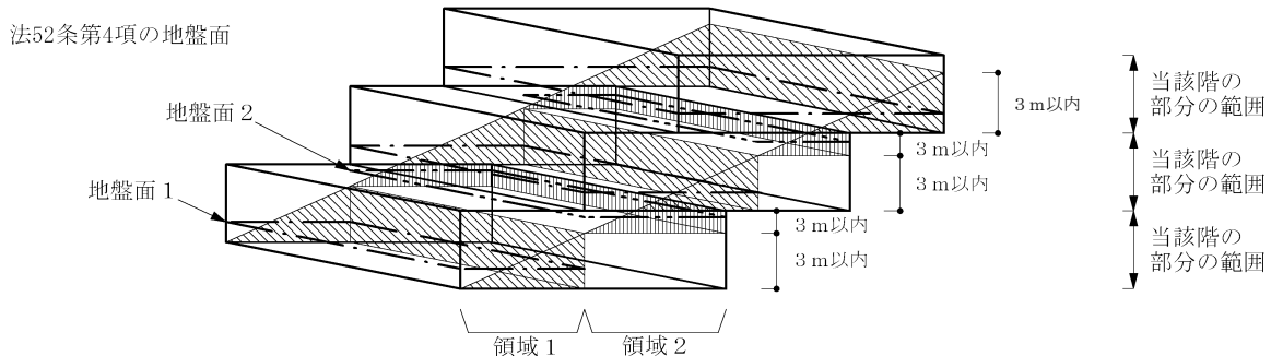
図 1 法 52 条第 4 項の地盤面
