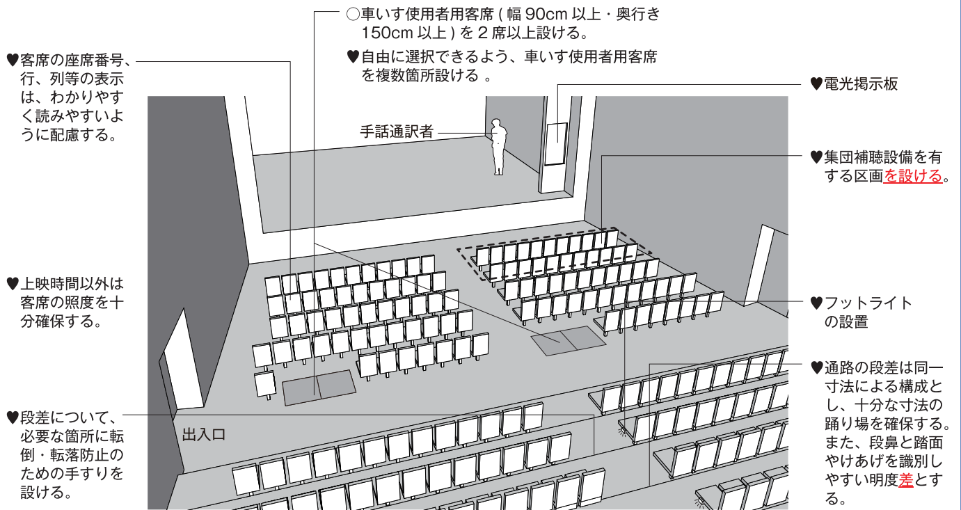
図12-1 客席の整備例
