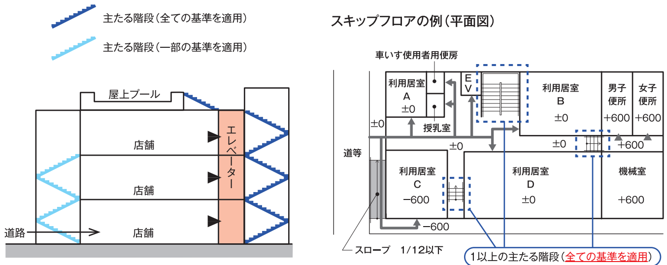
図 6-7 エレベーター等を設置した場合の整備基準の適用範囲
