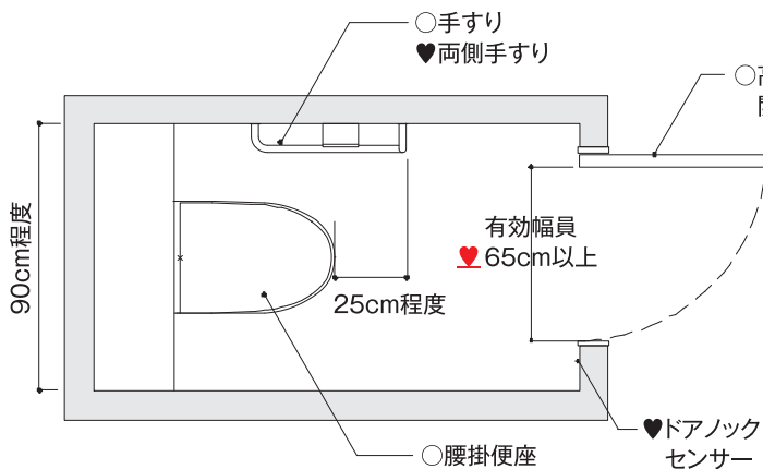
図9-4 その他の便房の例
