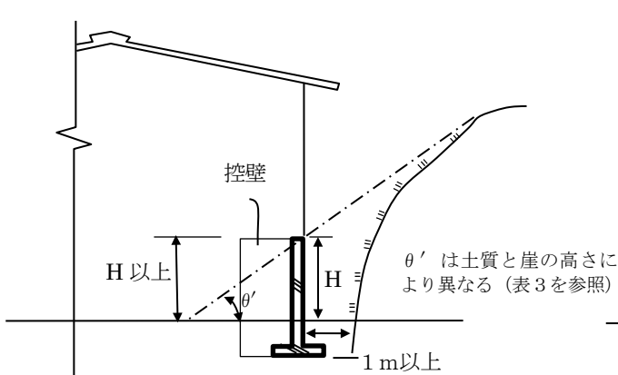
図 8 基礎の立上げ(布基礎)
