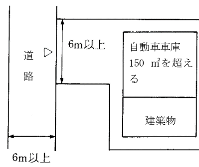
図3 自動車車庫の床面積の合計が150㎡超の場合
