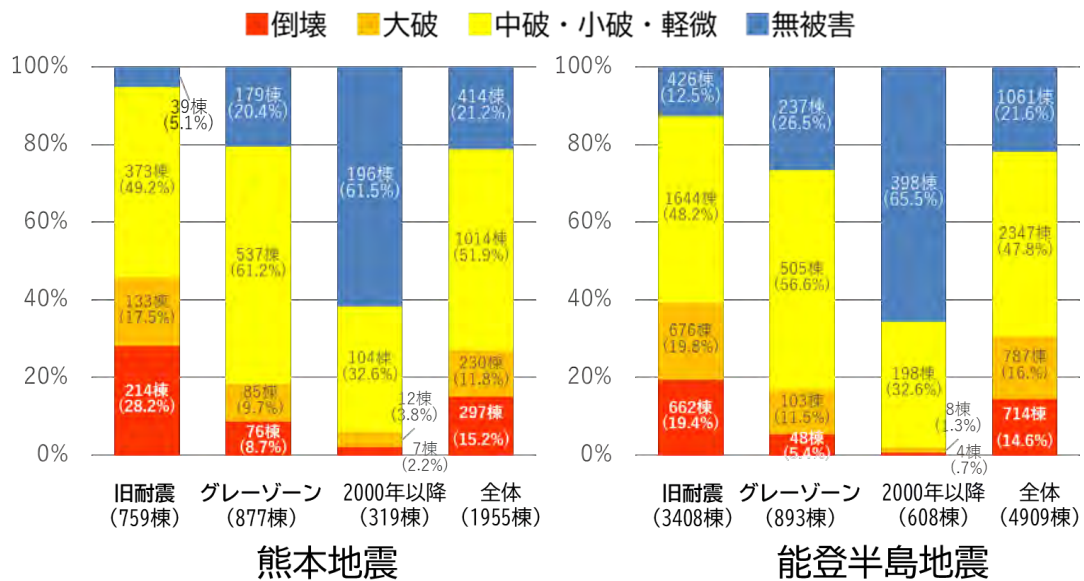
図 2-1-2 熊本地震における木造建築物の建築時期別の被害状況
