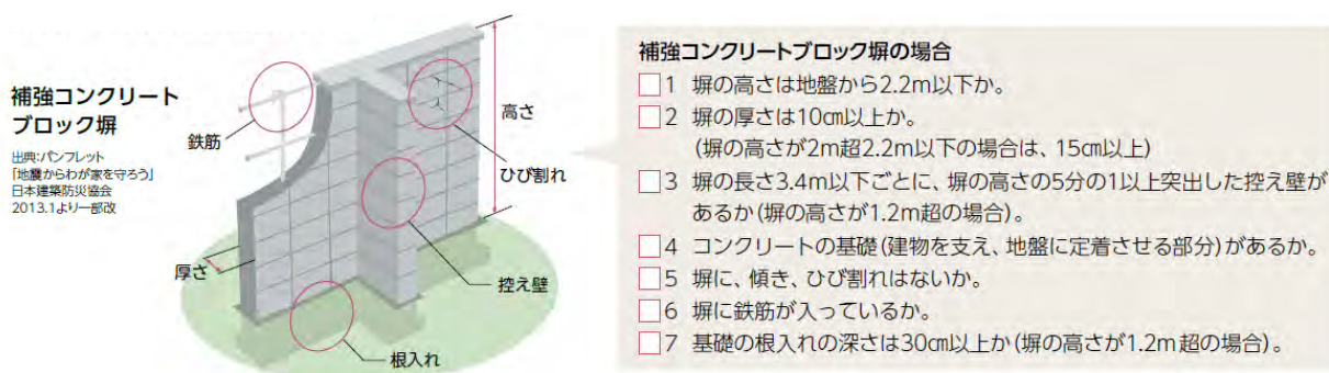
図3-2 補強コンクリートブロック塀の点検のチェックポイント（国土交通省HPより）
