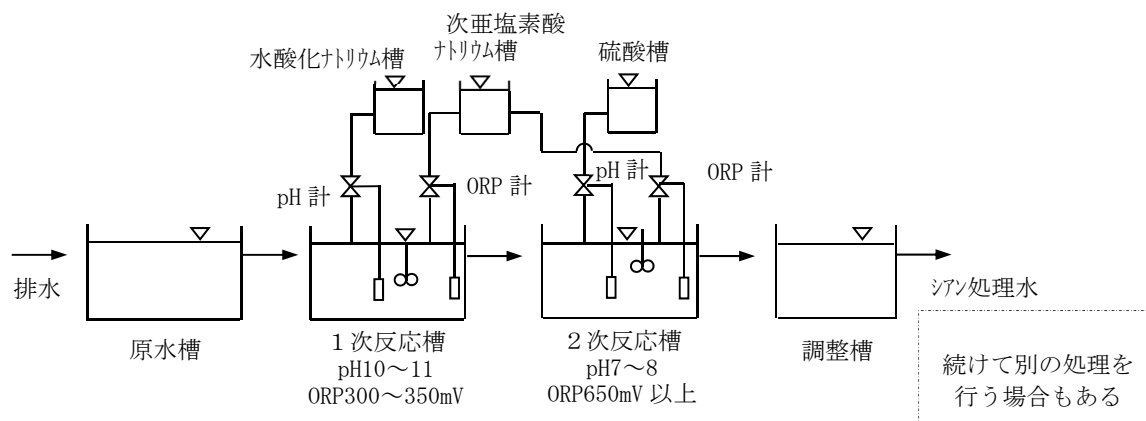
図ー 1 3 シアン含有排水の処理フロー(アルカリ塩素法)
