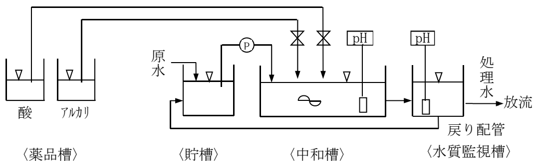
図－３ 中和法による一般的処理フロー
