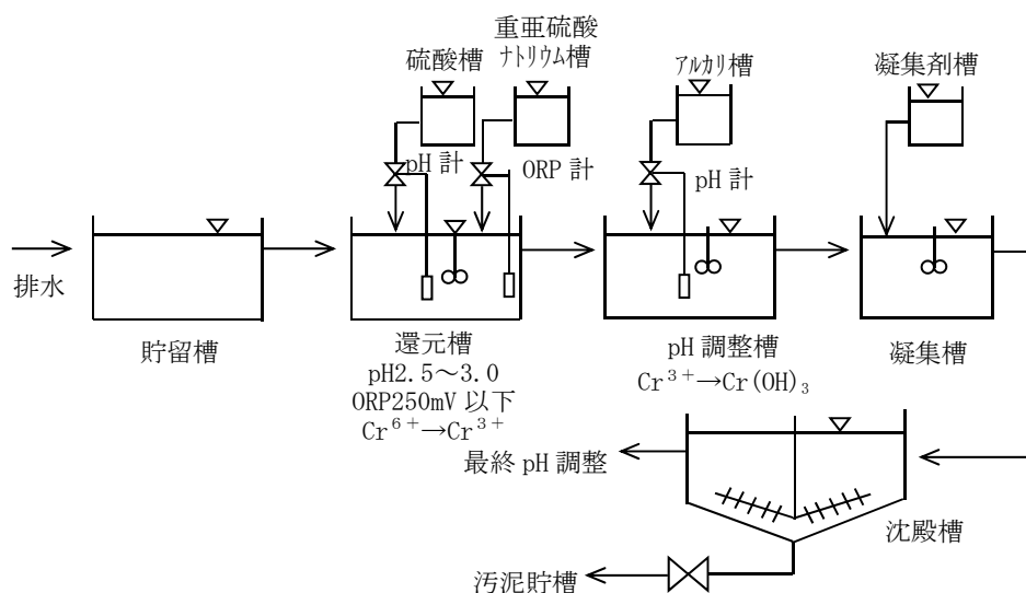
図－１２ 六価クロム処理フロー（還元法）
