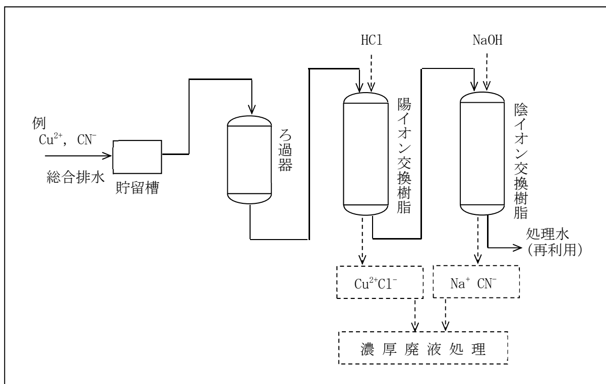
図－14 イオン交換法の概略図
