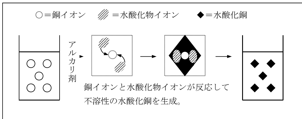
図－５ 不溶化の仕組み
