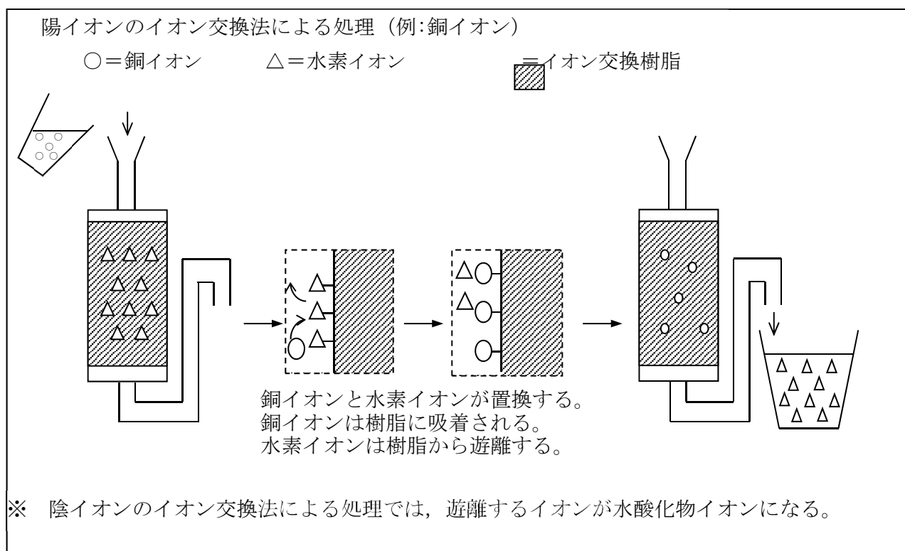
図－１５ 陽イオンのイオン交換法による処理
