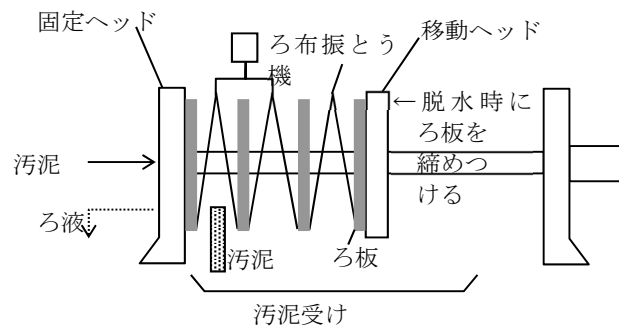
全 体 概 略 図
