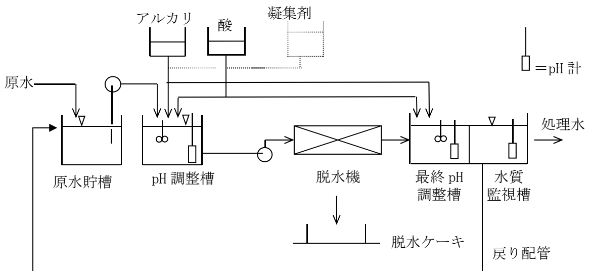
図－１１ 凝集・全量ろ過法の全フロー図
