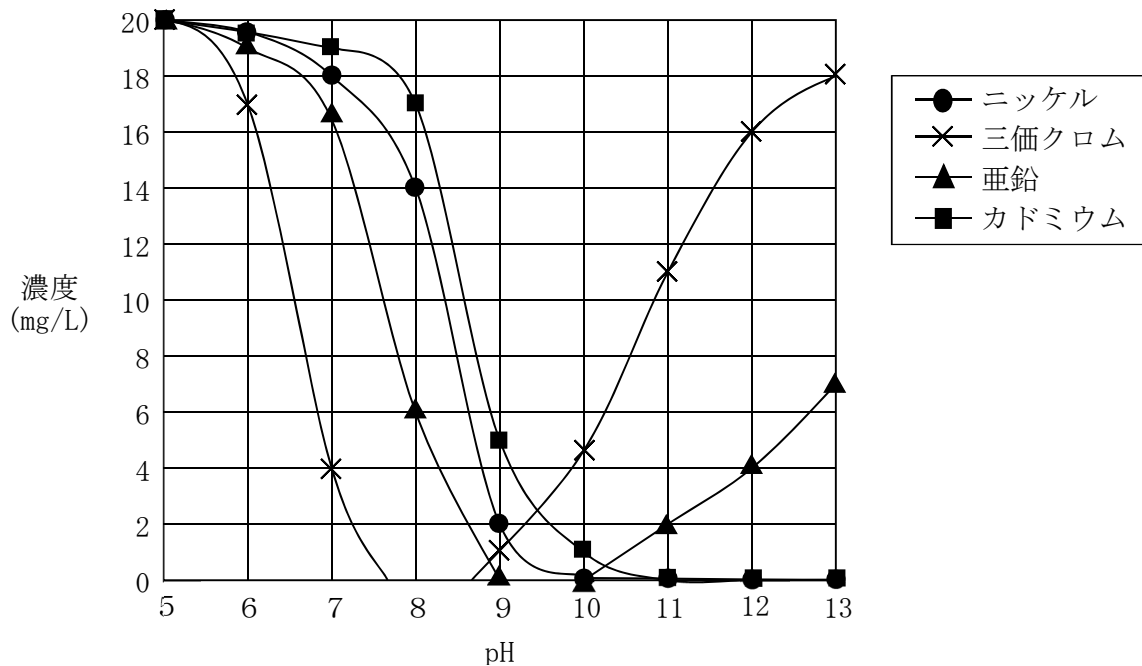
図－6 各種金属の濃度と pH の関係
