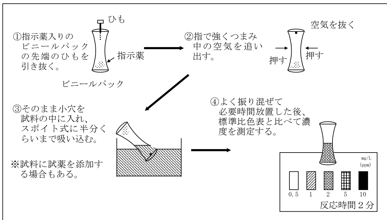
図－4 比色法の例（ビニールパック式）
