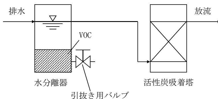
図－１８ 吸着法の一例
