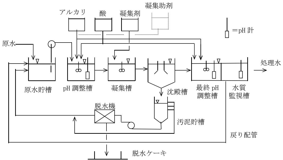
図－１０ 凝集沈殿法の全フロー
