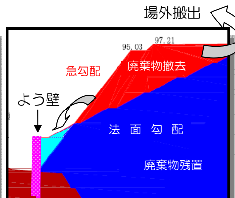
<処分場整形断面図>
