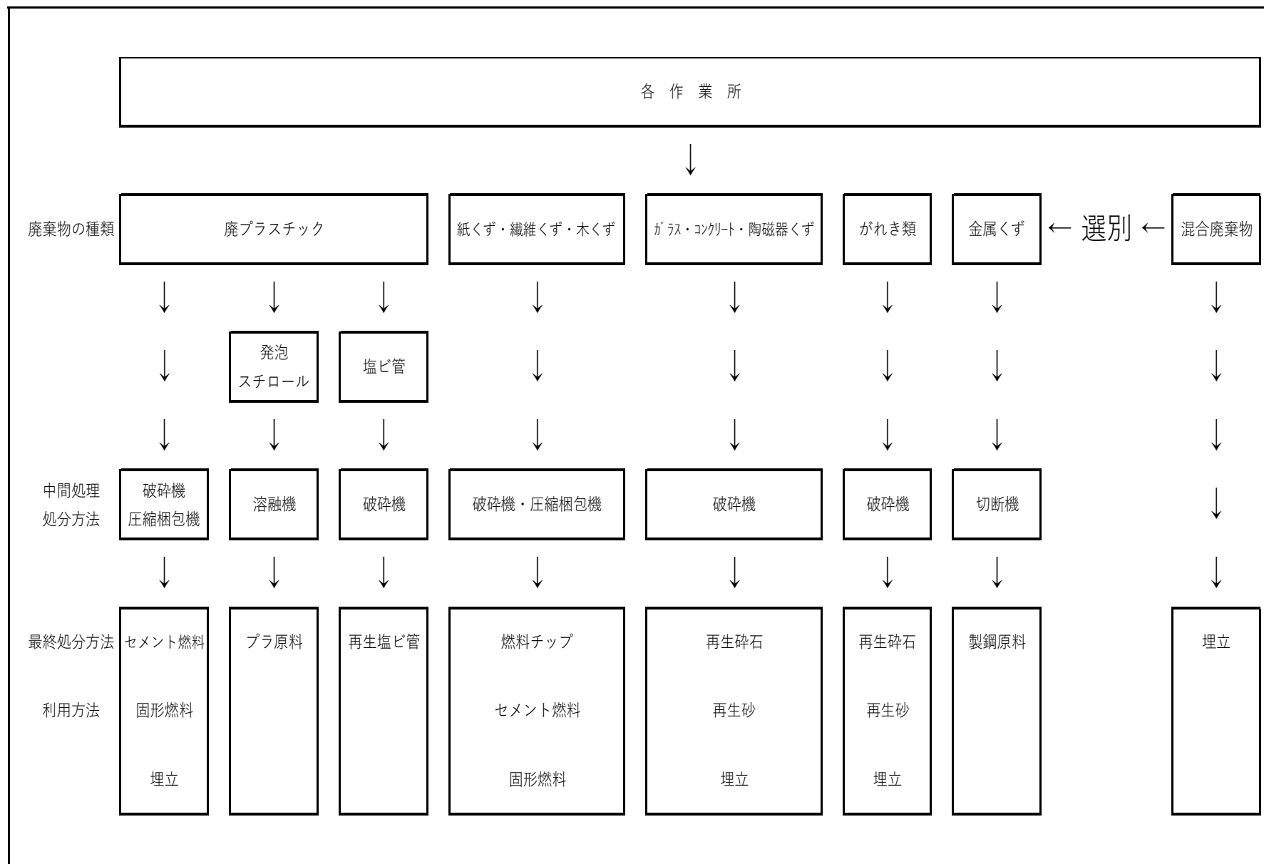
別添 1 処理工程図
