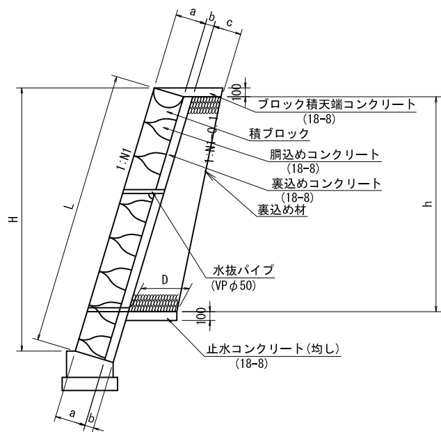
標準断面図
