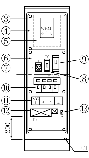
(参考内部図)
