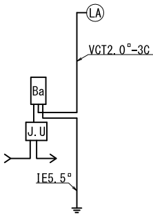
結線図
