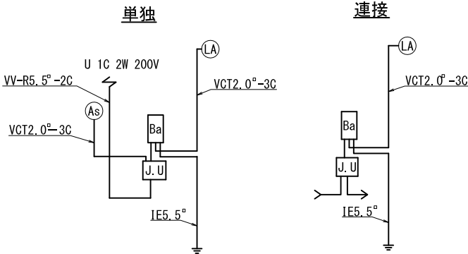
結線図
