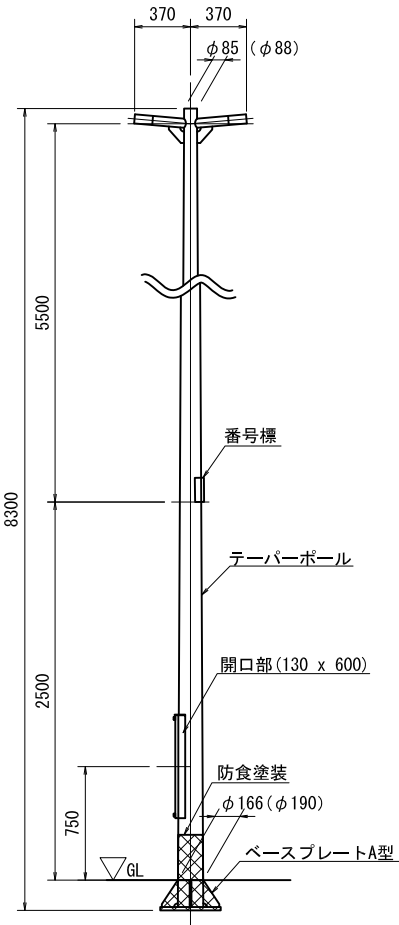
灯柱詳細図 S=1:50
