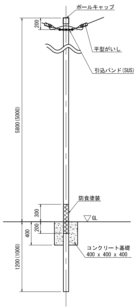
中間柱詳細図 S=1:40
