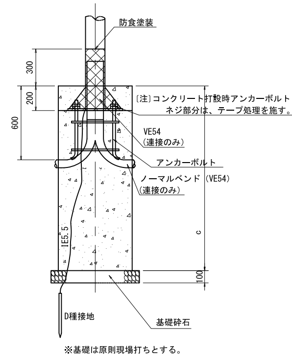
基礎詳細図
