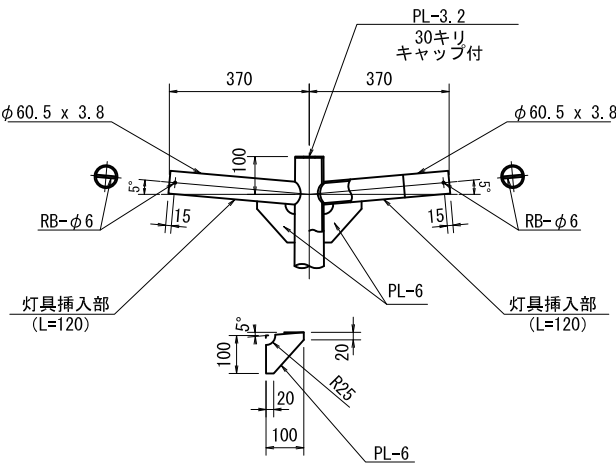
アダプター詳細図 S=1:20
