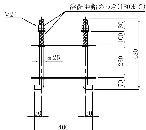
アンカーボルト 300×130 (Ac・Bolt B型)
