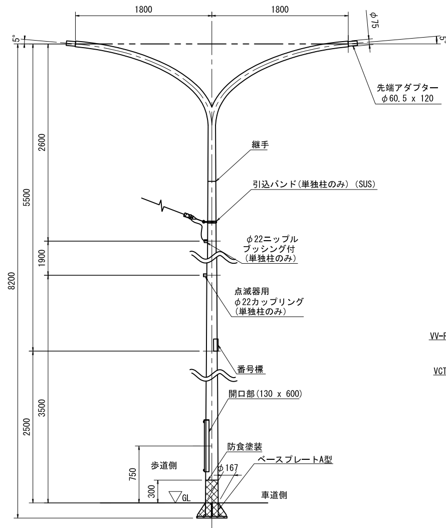
灯柱詳細図 S=1:50
