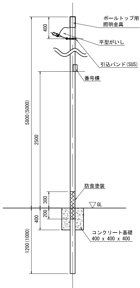
照明灯柱詳細図 S=1:40
