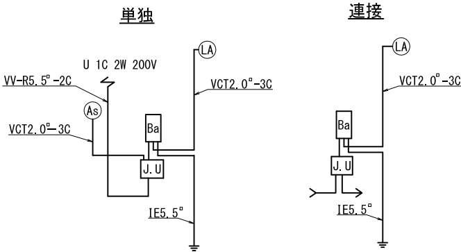
結線図
