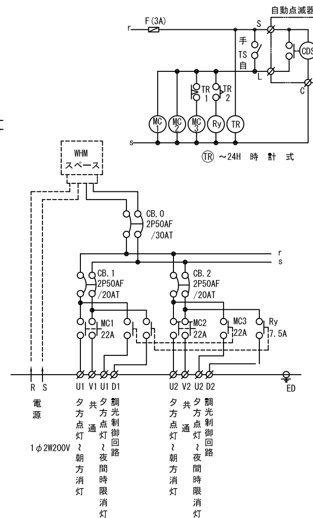
結線図
