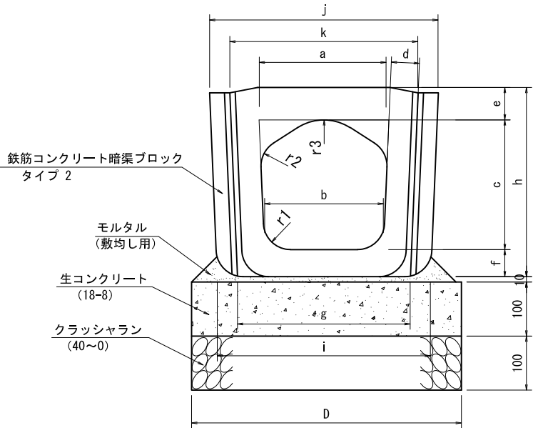
寸 法 表
