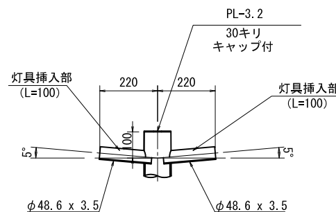
アダプター詳細図 S=1:20
