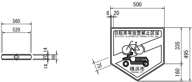
寸法及び材料表 (1基当り)
