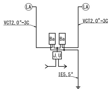
結線図
