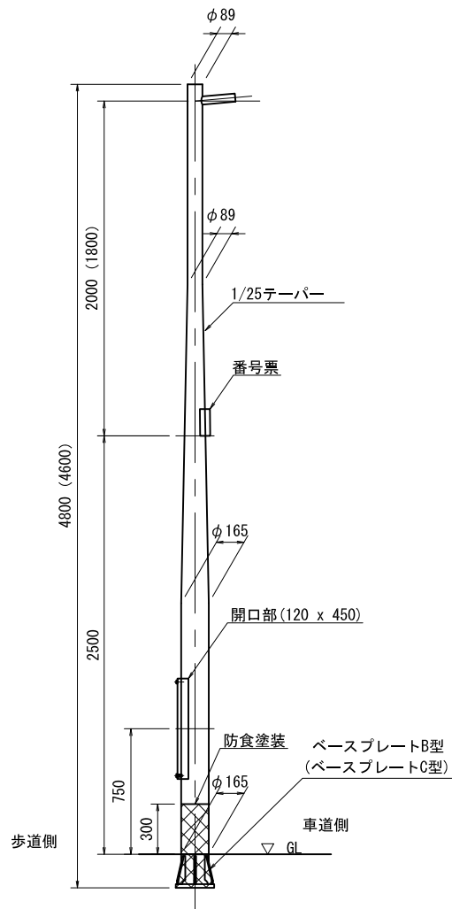
灯柱詳細図 S=1:40
