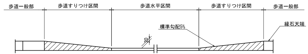
A-A' 展開図
