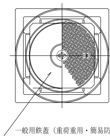
平面図
