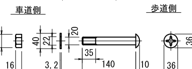
タイプA (M20 x 140)
