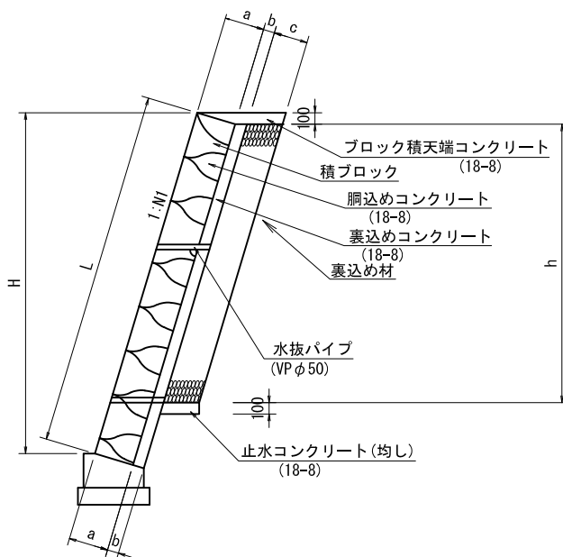
標準断面図
