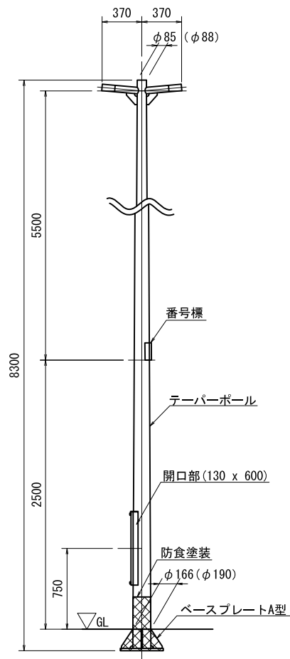
灯柱詳細図 S=1:50
