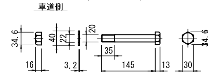
タイプB (M20 x 145)
