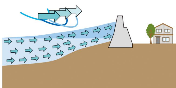
図-2 吹き寄せ効果 国土交通省「高潮発生のメカニズム」を元に作成 (https://www.mlit.go.jp/river/pamphlet_jre/kaigan/kaiganduku/takashio/1mecha/01-2.htm)
