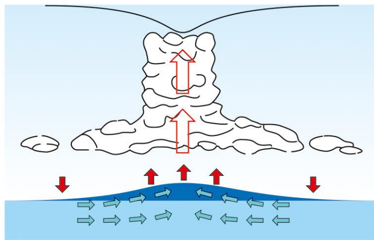
図-1 吸い上げ効果 国土交通省「高潮発生のメカニズム」を元に作成 (https://www.mlit.go.jp/river/pamphlet_jre/kaigan/kaigandukuri/takashio/1mecha/01-2.htm)
