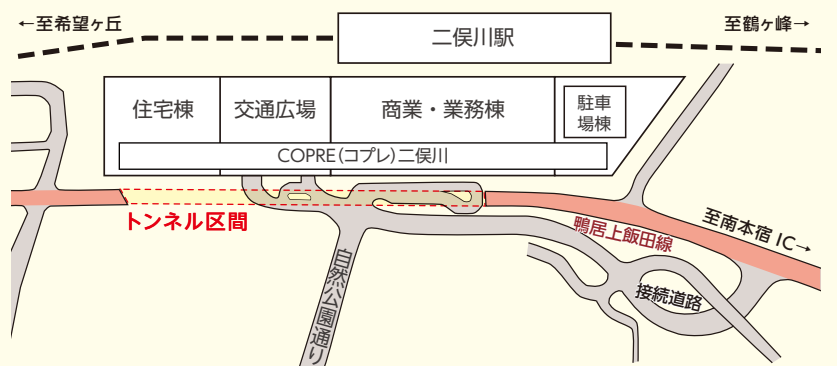
▲完成形平面図
