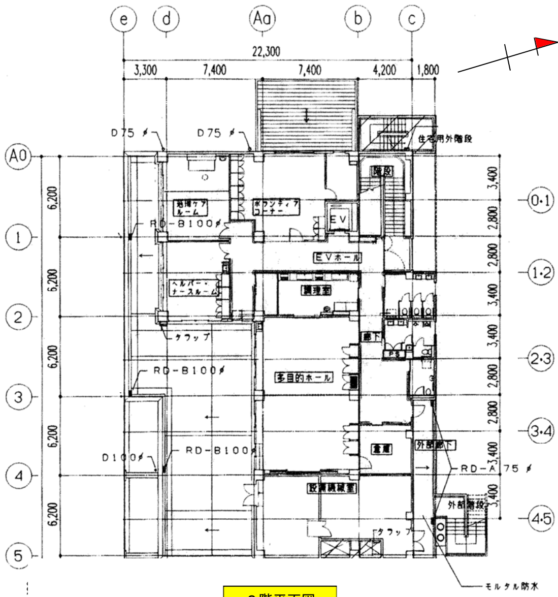
2階平面図
