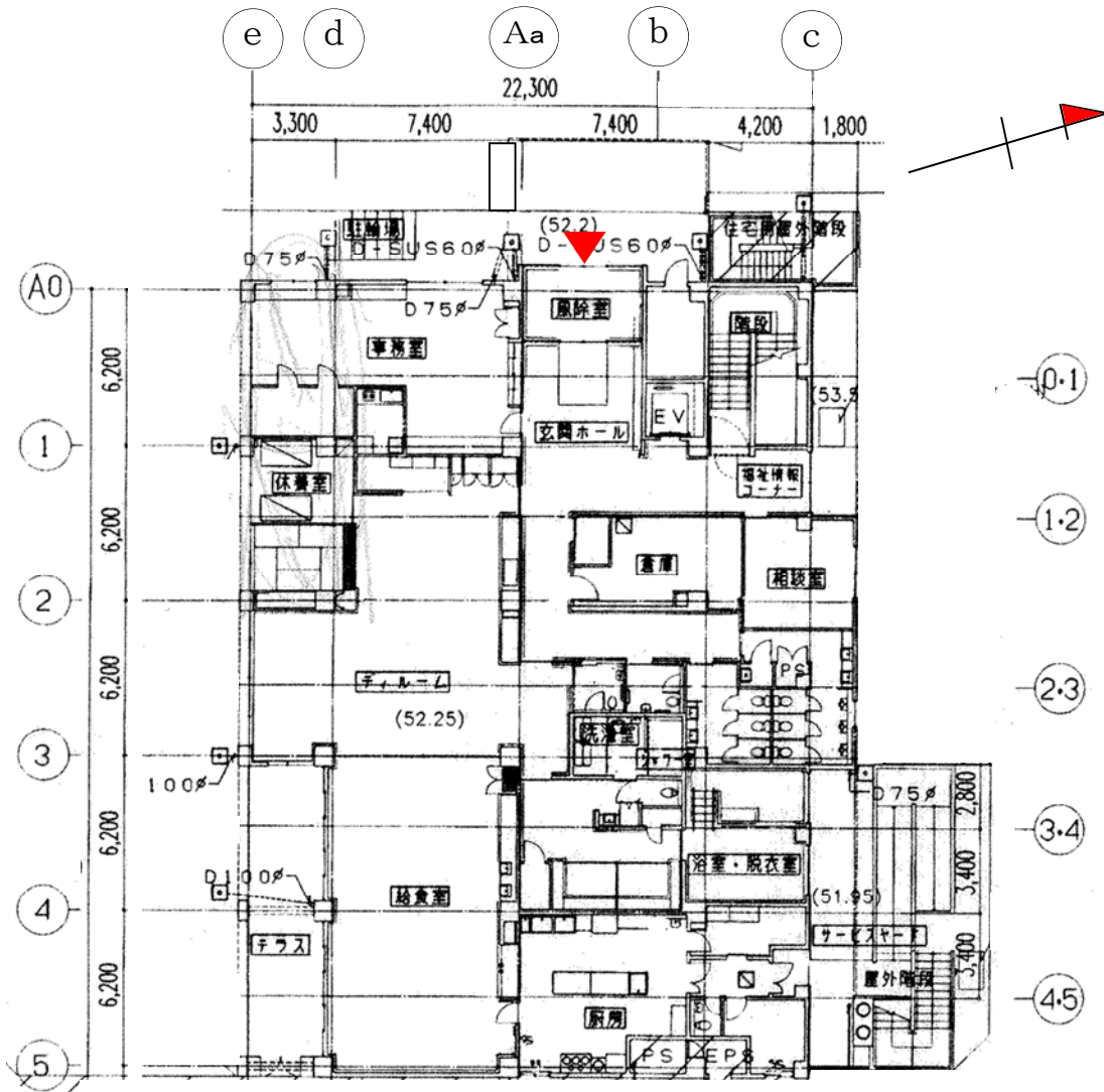
1階平面図
