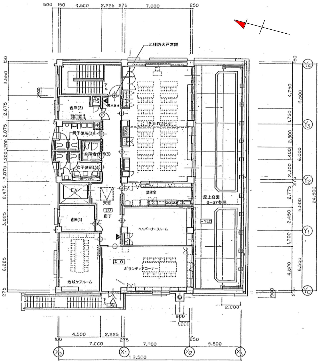
2階平面図
