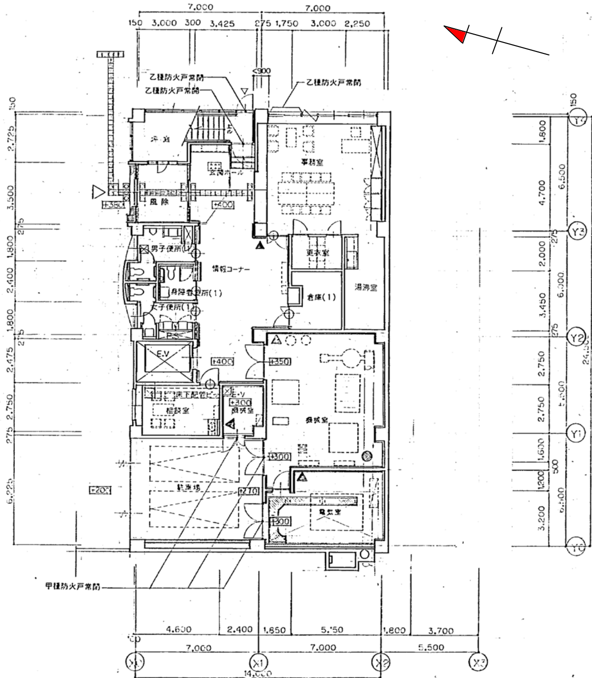
地下1階平面図
