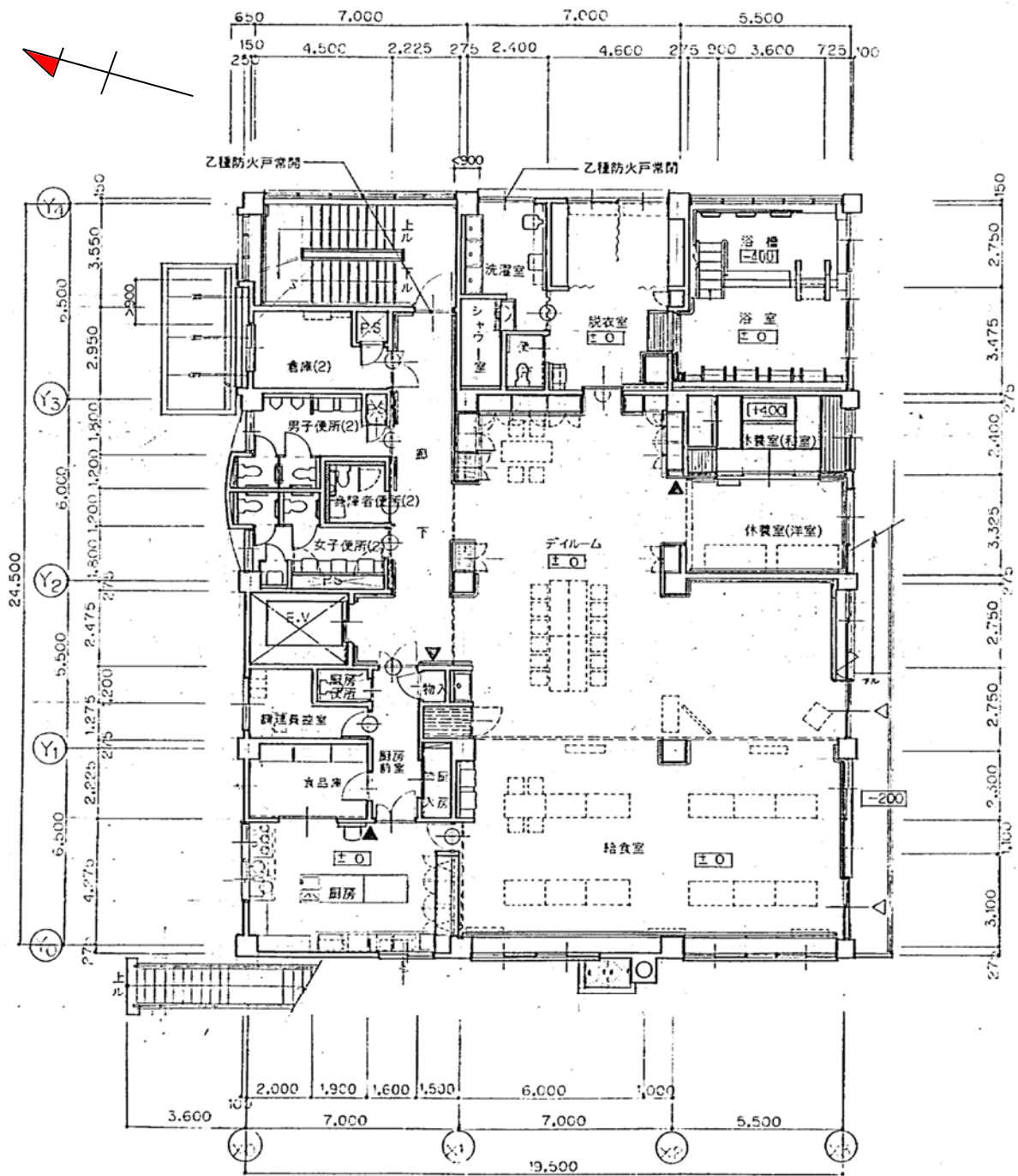
1階平面図
