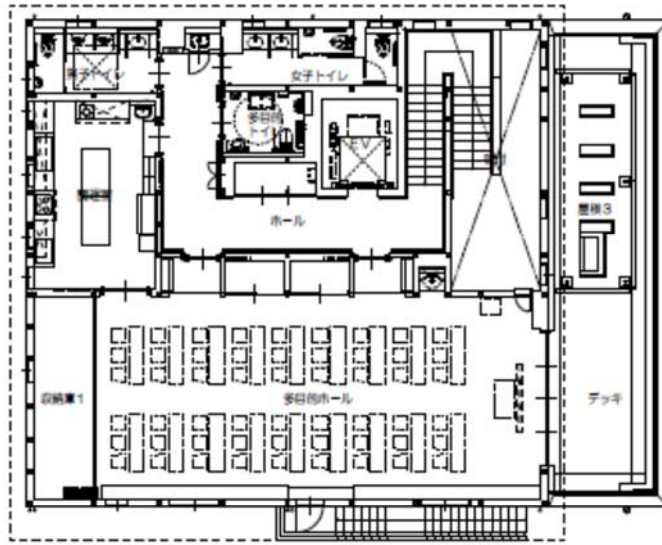
2階平面図 1/100
