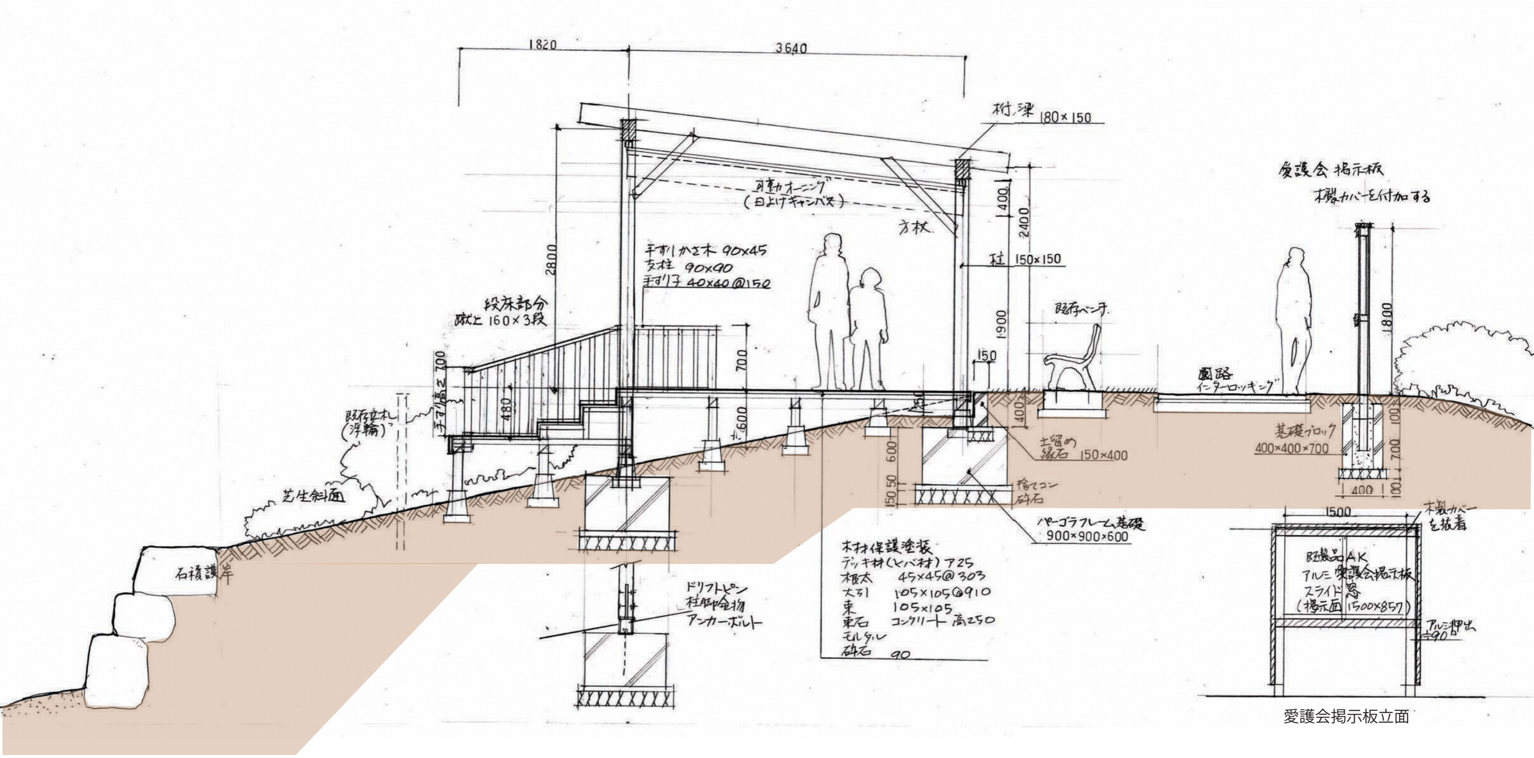
断面図 1:40
