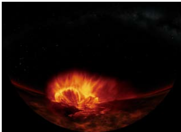
▲オーロラ発生メカニズム・アニメーション ©GOTO, E&S
