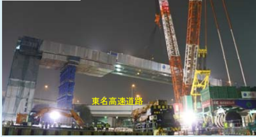
①横浜青葉IC・JCT付近 上部工架設(H29.10.11東名通行止め) ※首都高施工区間
