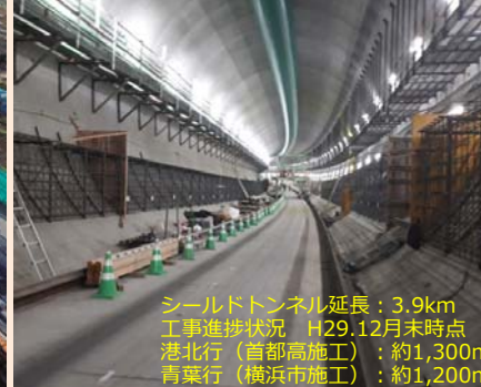
⑥シールド坑内
